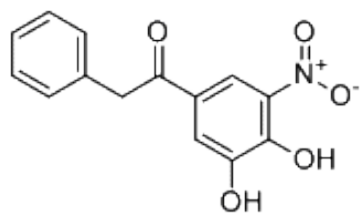
PC-3579101, DMSO-d6
